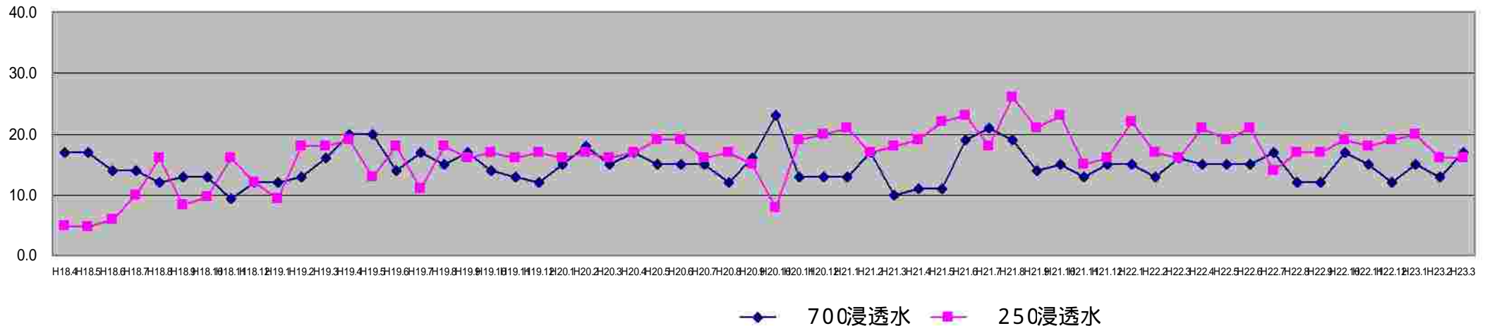
善和処分場水質推移 COD (mg/?)
